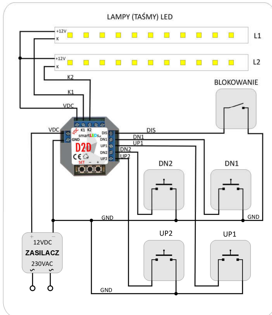
Rys. 3 Podstawowy schemat instalacji sterownika D2D (pełna regulacja jasności).
