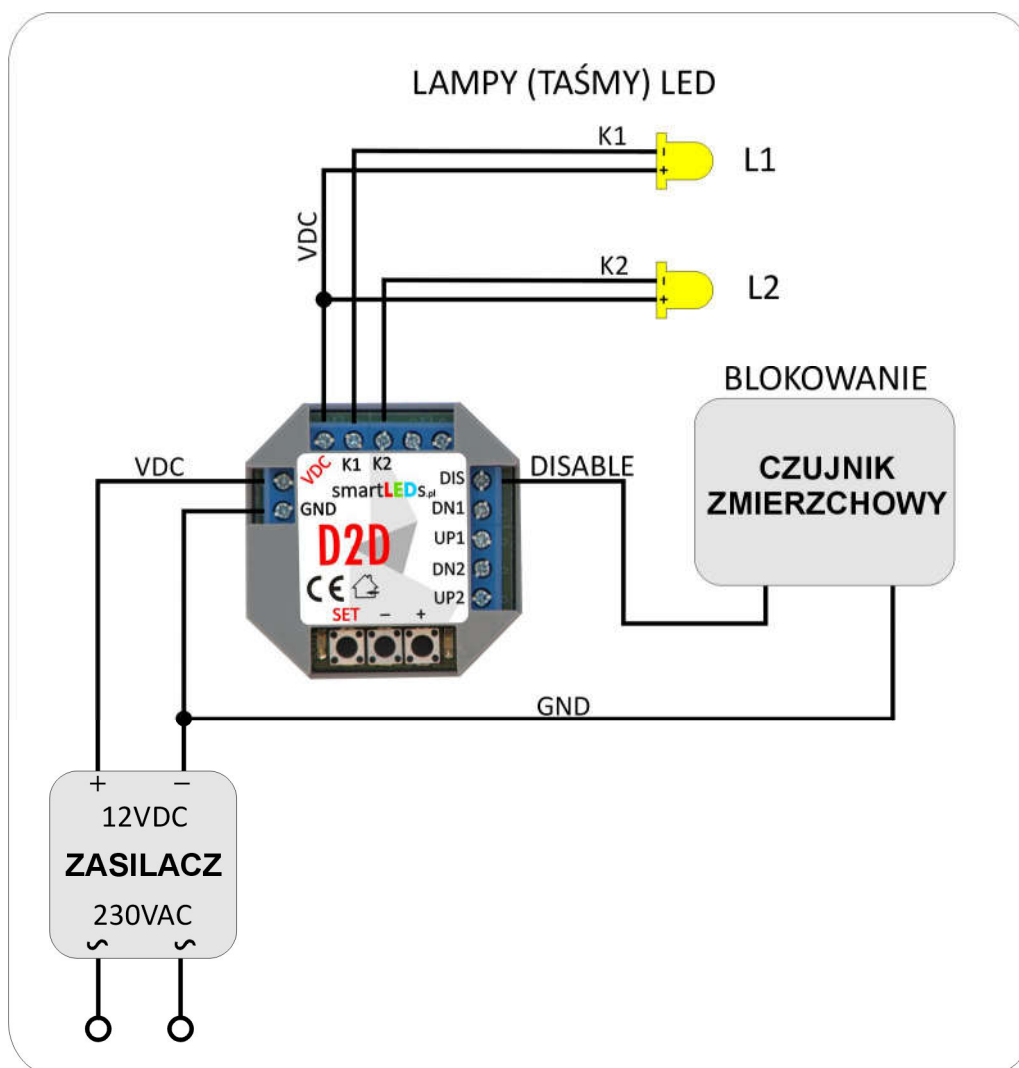
Rys. 4. Schemat uproszczonej instalacji do oświetlenia o stałej, wstępnie ustalonej jasności
