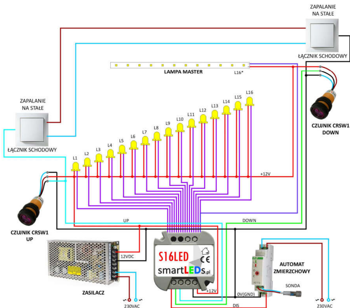
Rys. 4 Przykładowy schemat instalacji schodowej ze wspólnym zasilaczem Sterownika, czujników schodowych CRSW1 i lamp, z lampą Master, ze sterowaniem za pomocą czujników schodowych CRSW1, z funkcją zapalania lamp na stałe
