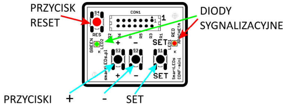
Rys. 2 Konfigurator CONFIG-mini
